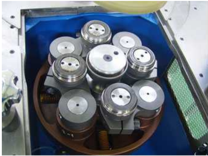
封罐轮
