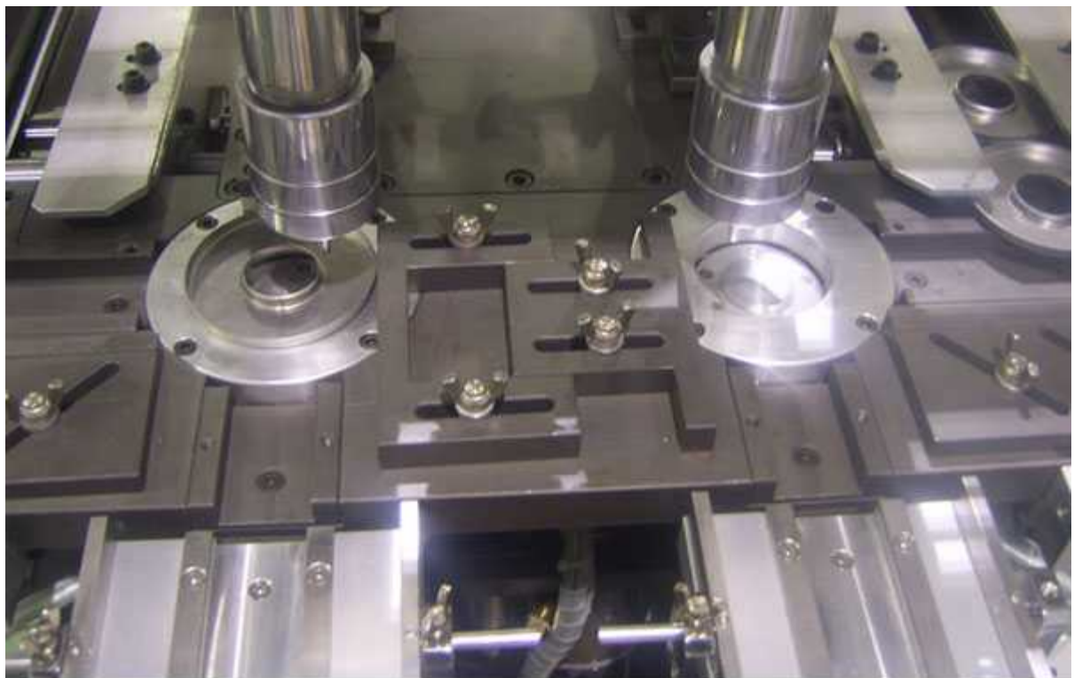
单组份注胶枪
