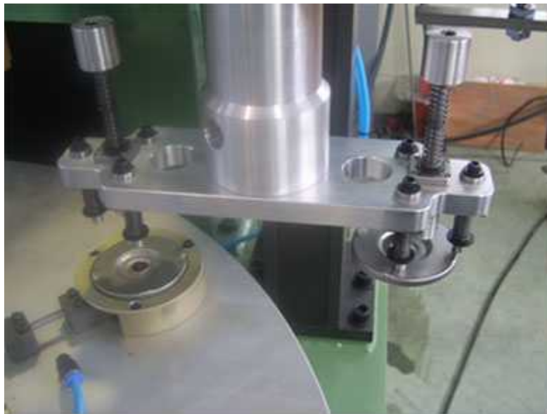
已碰焊的端盖及安全阀卸件
